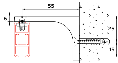
wandmontage met muurbeugel 4140
