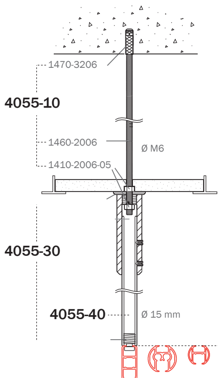
- plafondmontage 4100, 5100 of 4200 aan pendel 4055-40 met montageset 4055-30, pendel aan draadeindset 4055-10.
