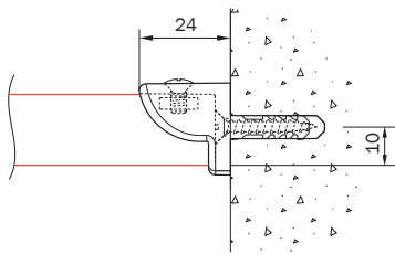
wandmontage 4200 met dagsteun 4249
