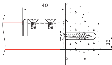
wandmontage 5100 met dagsteun 5149
