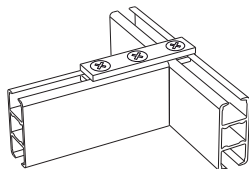
railverbinder 4130 als haakse verbinder
