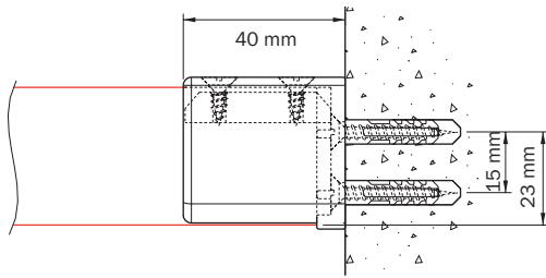
wandmontage 4100 met dagsteun 4149
