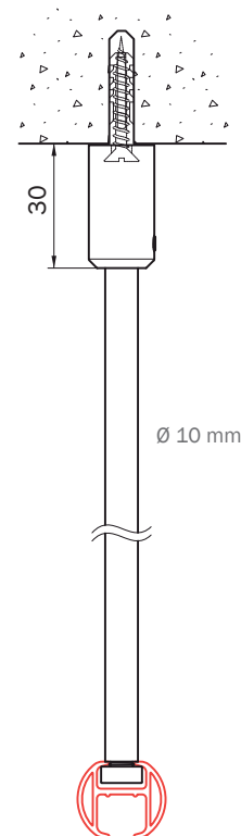
plafondmontage met 4255
