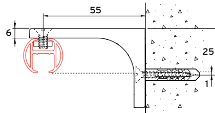
montage 4200 met muurbeugel 5140
