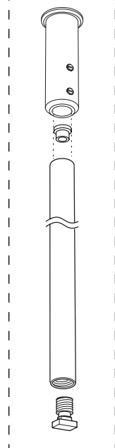
4055-30 diverse montagesets inclusief plafondklos ook sets voor NEN1010
