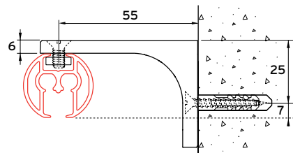
montage 5100 met muurbeugel 5140
