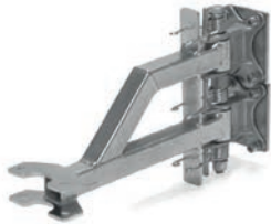
Basisdeel HD-haak 90° (verlaagd) Artikel Nr H7070
